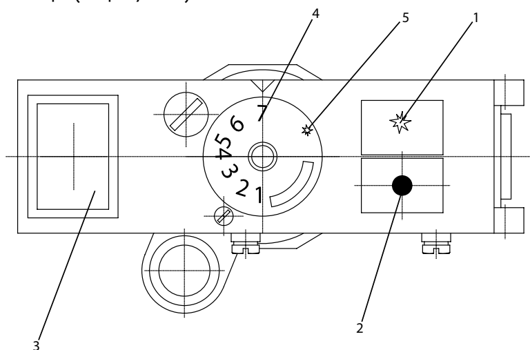
Рисунок 2 — Блок газовый
